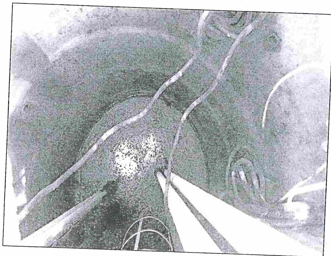
Szennyvíz átemelő szivattyúk felújítása
