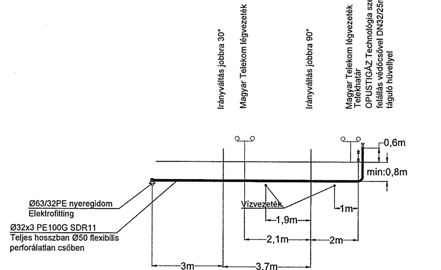
Hosszszelvény M 1:100
